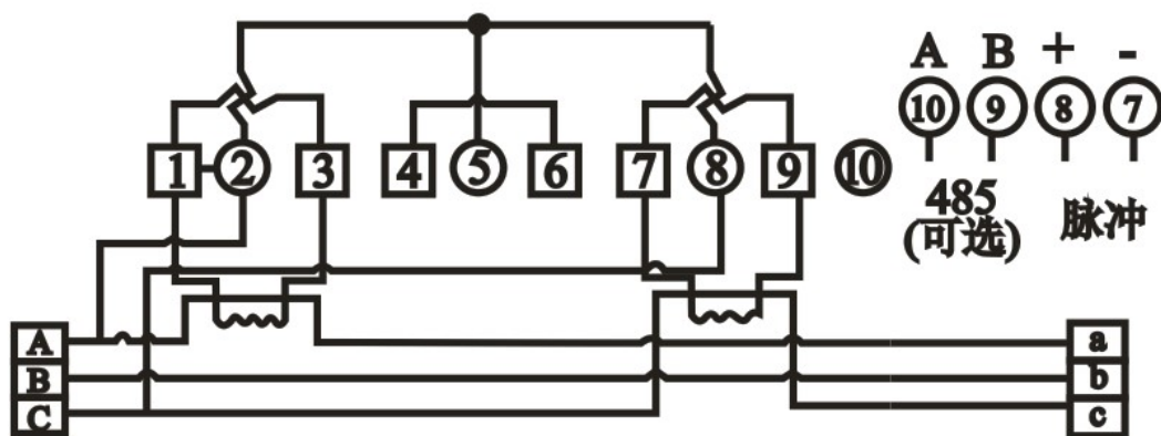
三相三线互感式接线图
