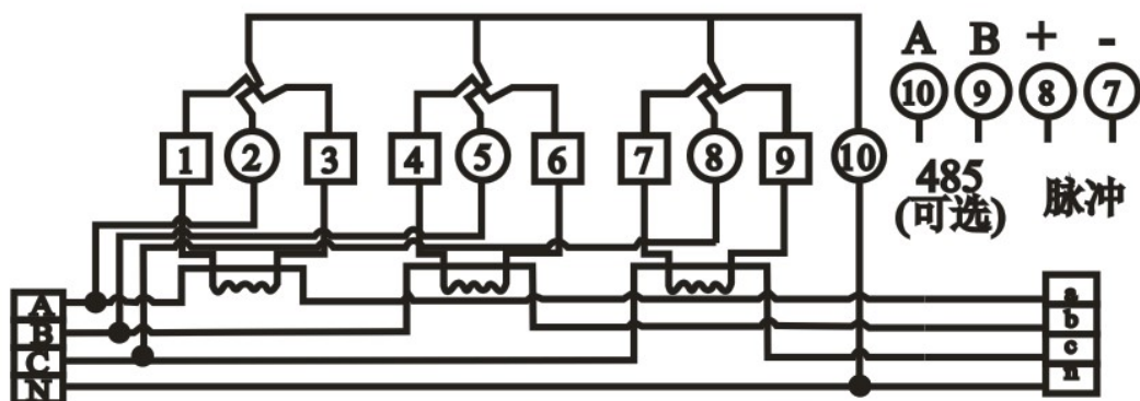
三相四线互感式接线图
