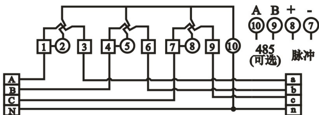
三相四线直接式接线图
