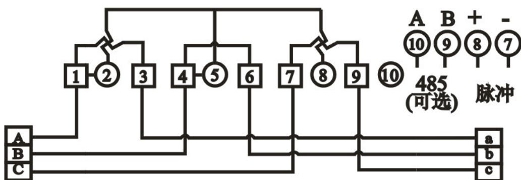
三相三线直接式接线图
